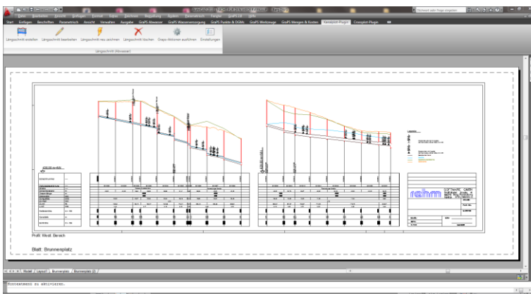
KANALPLOT-Plugin: Kanallängsschnitt (Details siehe Programm KANALPLOT )
